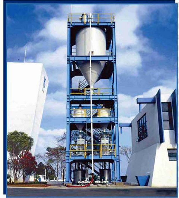
🔹 Sistemas de Estocagem e Dosagem de Cal
